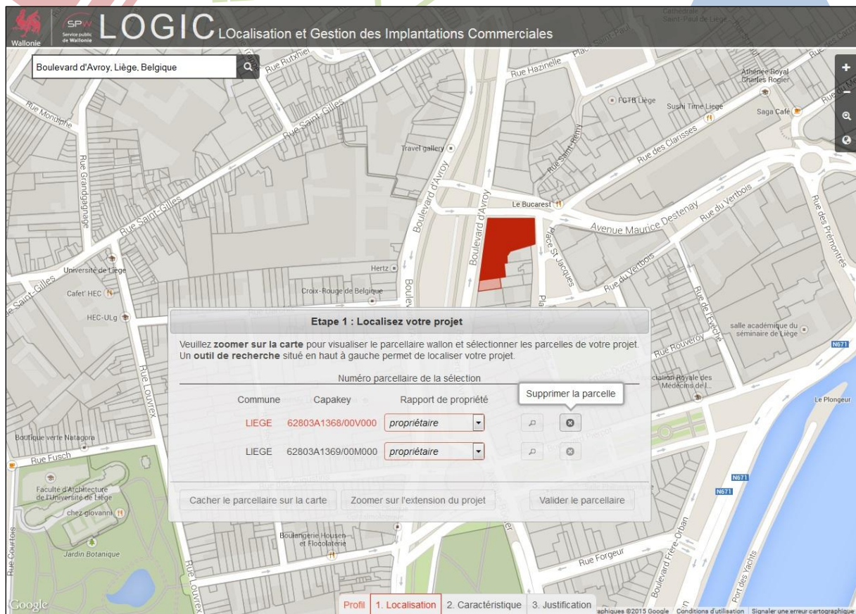
Figure 13. Interaction entre la fenêtre amovible et la carte
